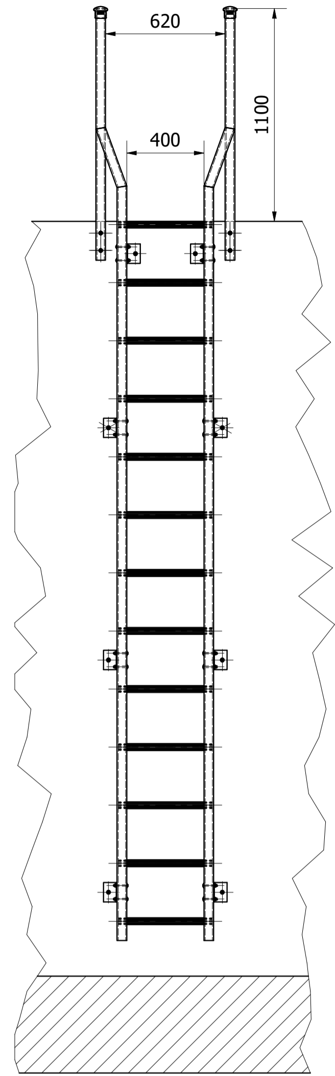
ŽEBŘÍK S ČELNÍM VÝSTUPEM
