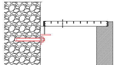
Konzola pro 2-dílné rošty
