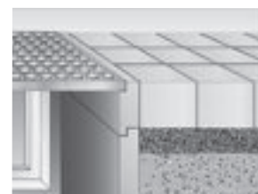
Betonový nástavec MEAVECTOR - schema
