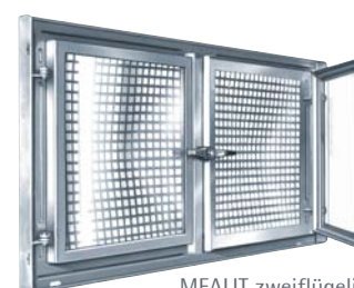
MEALIT zweiflügelig
