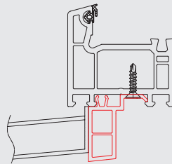
Querschnitt Einbau FBA 30
