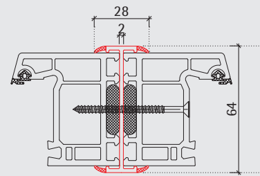
Einbau-Beispiel Kopplung Typ H
