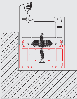
Querschnitt Einbau BRV 30
